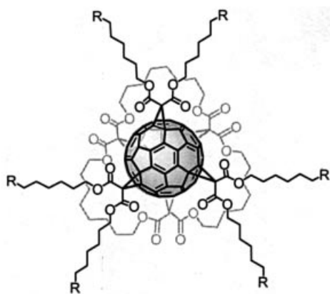
25 R = -NH-Boc
